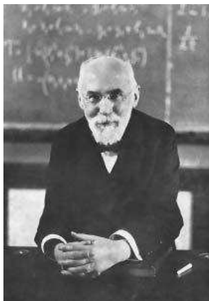
Хендрик Лоренц (1853-1928), дански физичар, добитник Нобелове награде 1902.
