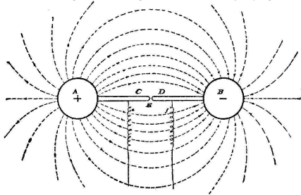
Херцов осцилатор
